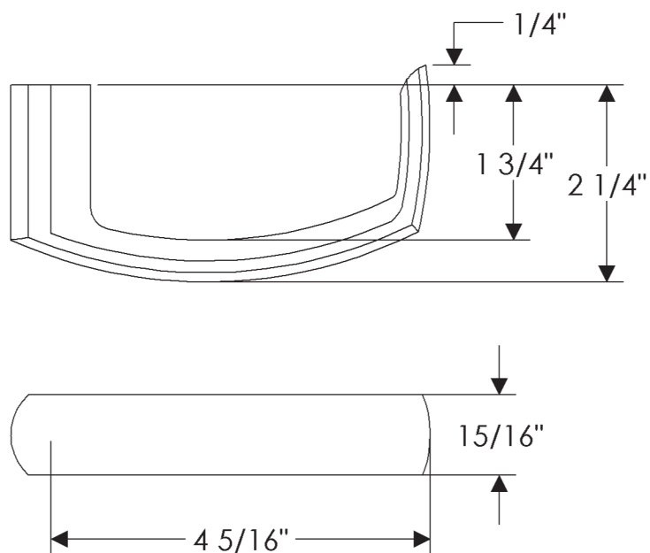
L314 UJ Return Lever
